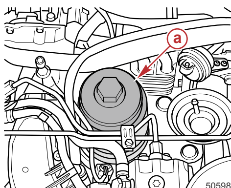
a - Ölfilterdeckel
